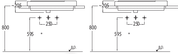
VERDA Washbasin (75 cm.)
